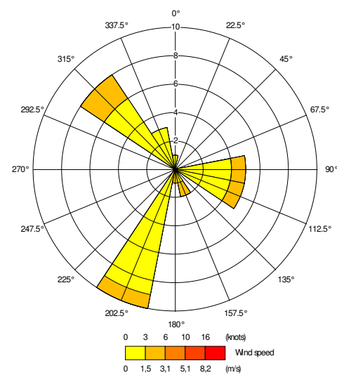
Profilo anemometrico orario medio postazione via Rizzoli - ore 18:00
