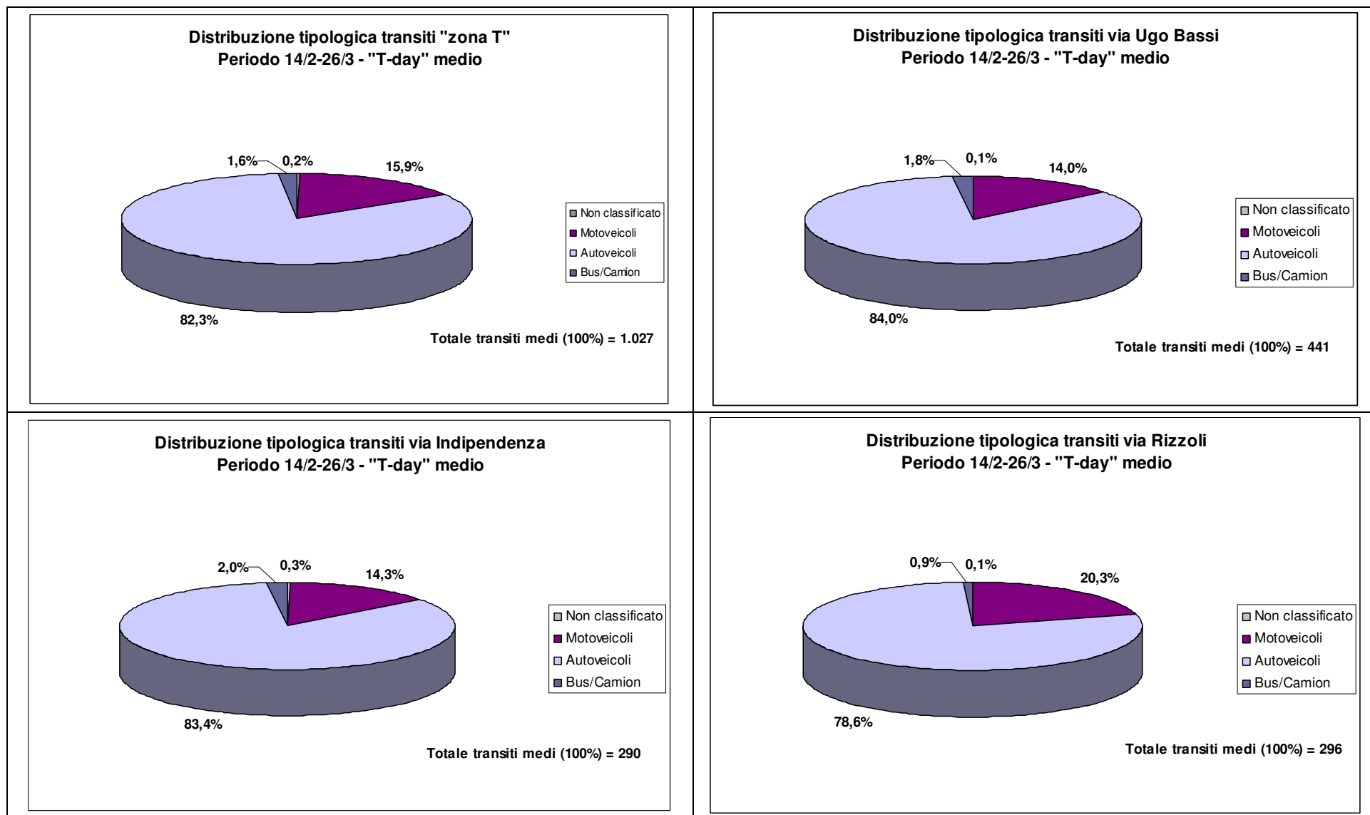
Figura A.4.1 – Distribuzioni per tipologie di veicolo dei transiti registrati nella "zona T" nella giornata "T-day" medio.
