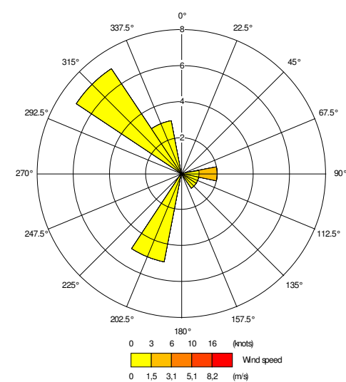
Profilo anemometrico giornaliero postazione via Rizzoli - giorno 8/3
