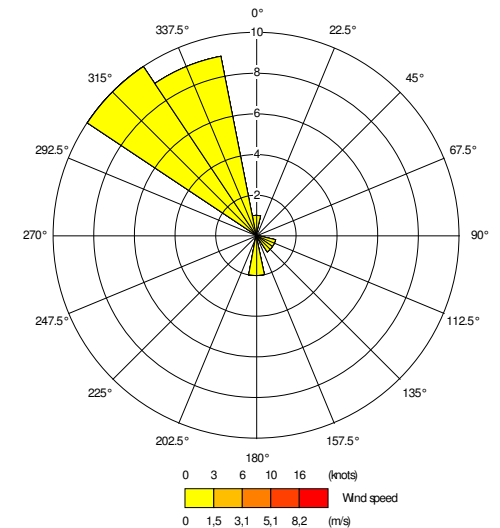
Profilo anemometrico giornaliero postazione via Rizzoli - giorno 26/3
