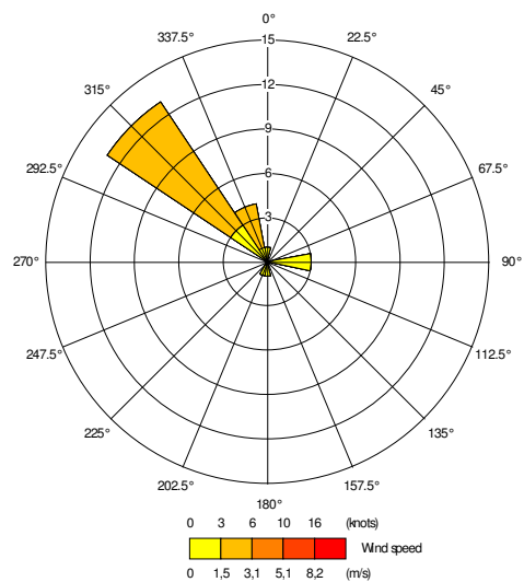
Profilo anemometrico giornaliero postazione via Rizzoli - giorno 18/3
