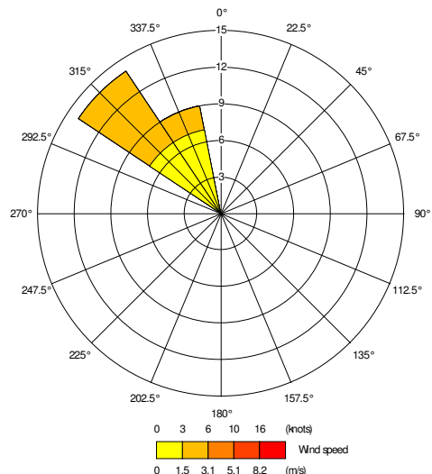
Profilo anemometrico giornaliero postazione via Rizzoli - giorno 1/3
