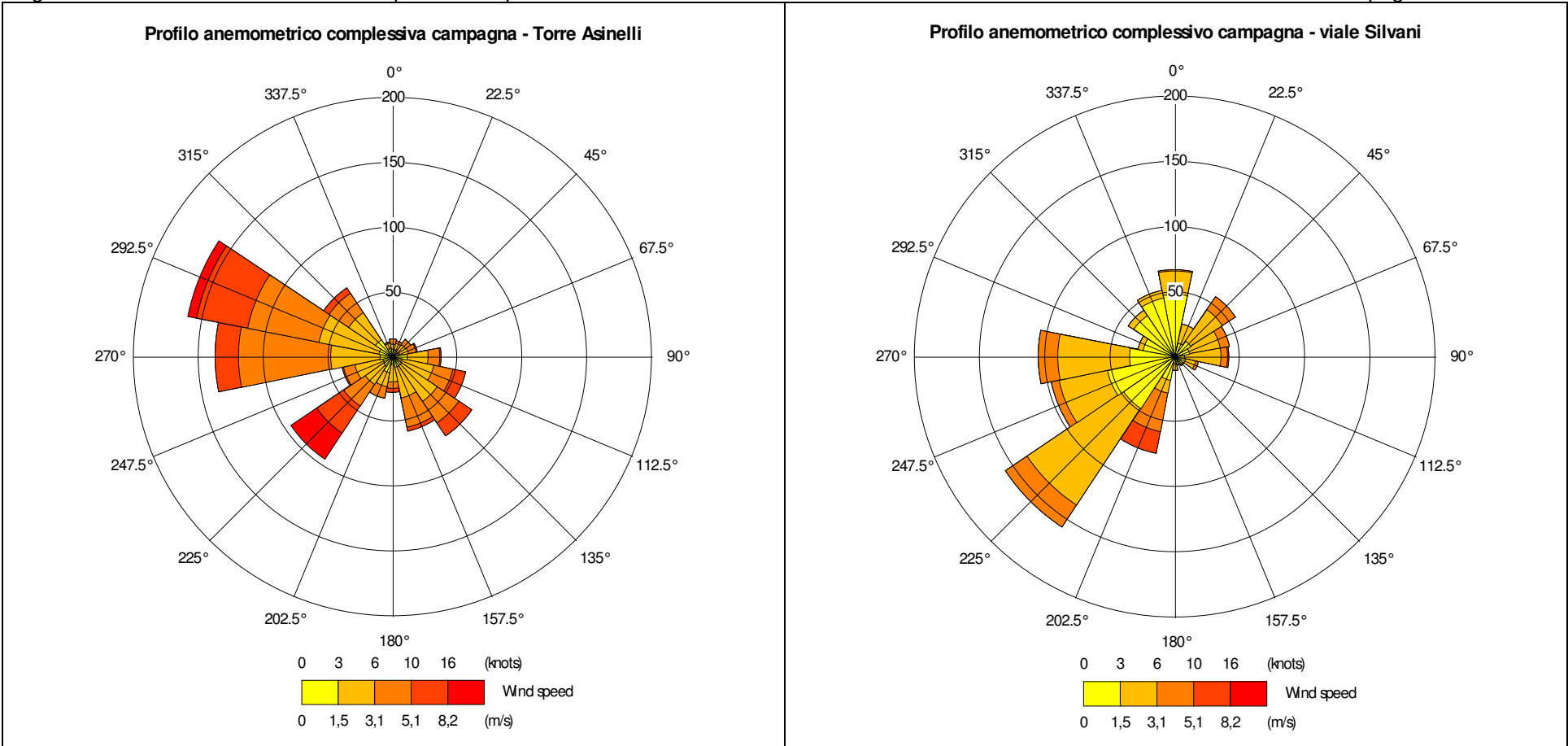
Figura A.3.3 – Profili anemometrici complessivi del periodo rilevati dalle stazioni di misura della Torre Asinelli e di viale Silvani durante la campagna
