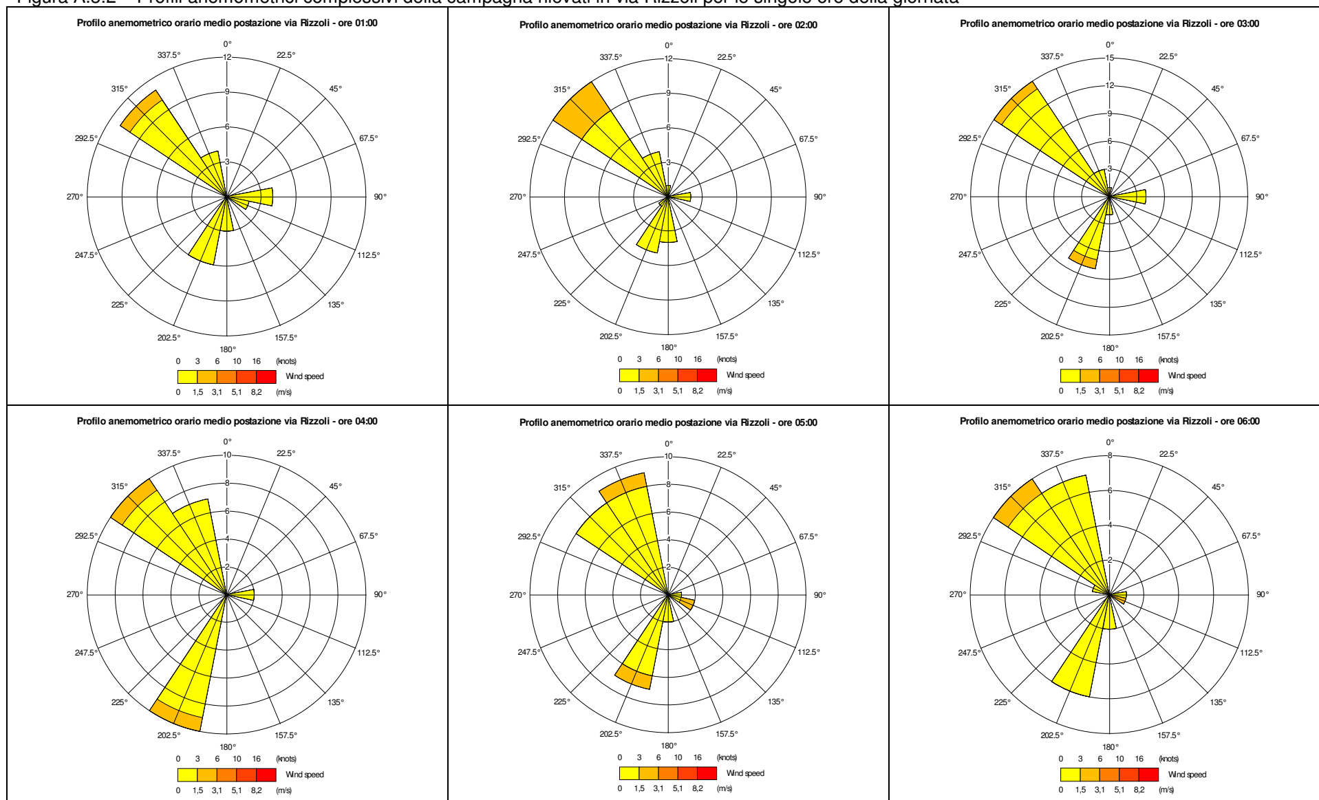
Figura A.3.2 – Profili anemometrici complessivi della campagna rilevati in via Rizzoli per le singole ore della giornata
