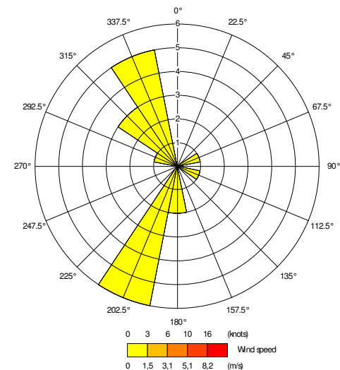
Profilo anemometrico giornaliero postazione via Rizzoli - giorno 14/3
