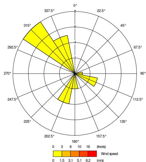
Profilo anemometrico giornaliero postazione via Rizzoli - giorno 12/3
