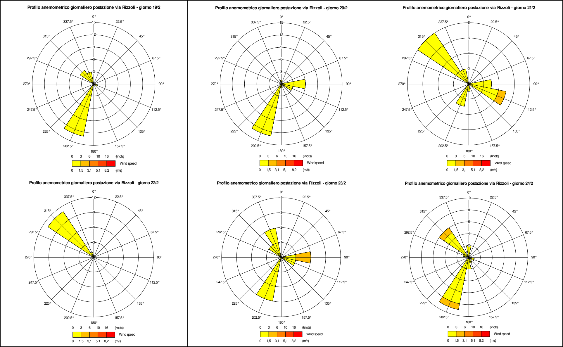
Figura A.3.1 – Profili anemometrici rilevati in via Rizzoli per le singole giornate di campagna
