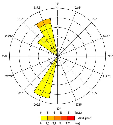
Profilo anemometrico giornaliero postazione via Rizzoli - giorno 28/2
