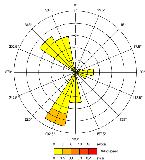
Profilo anemometrico orario medio postazione via Rizzoli - ore 00:00
