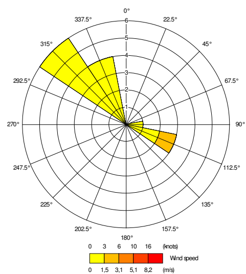
Profilo anemometrico giornaliero postazione via Rizzoli - giorno 6/3
