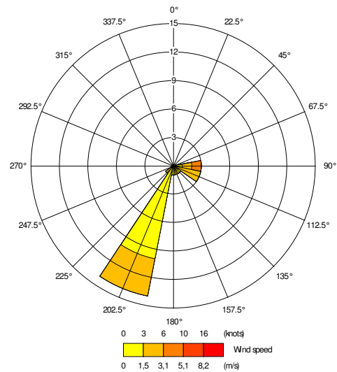
Profilo anemometrico giornaliero postazione via Rizzoli - giorno 19/3
