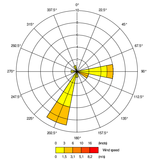
Profilo anemometrico giornaliero postazione via Rizzoli - giorno 20/3
