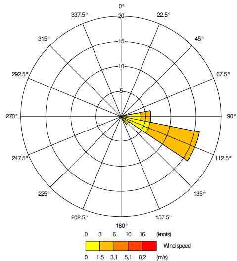
Profilo anemometrico giornaliero postazione via Rizzoli - giorno 24/3
