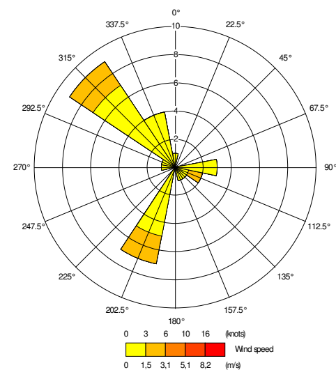
Profilo anemometrico orario medio postazione via Rizzoli - ore 12:00
