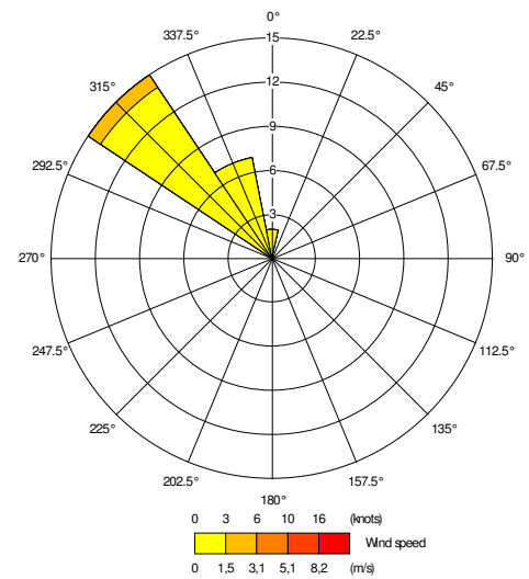
Profilo anemometrico giornaliero postazione via Rizzoli - giorno 25/3
