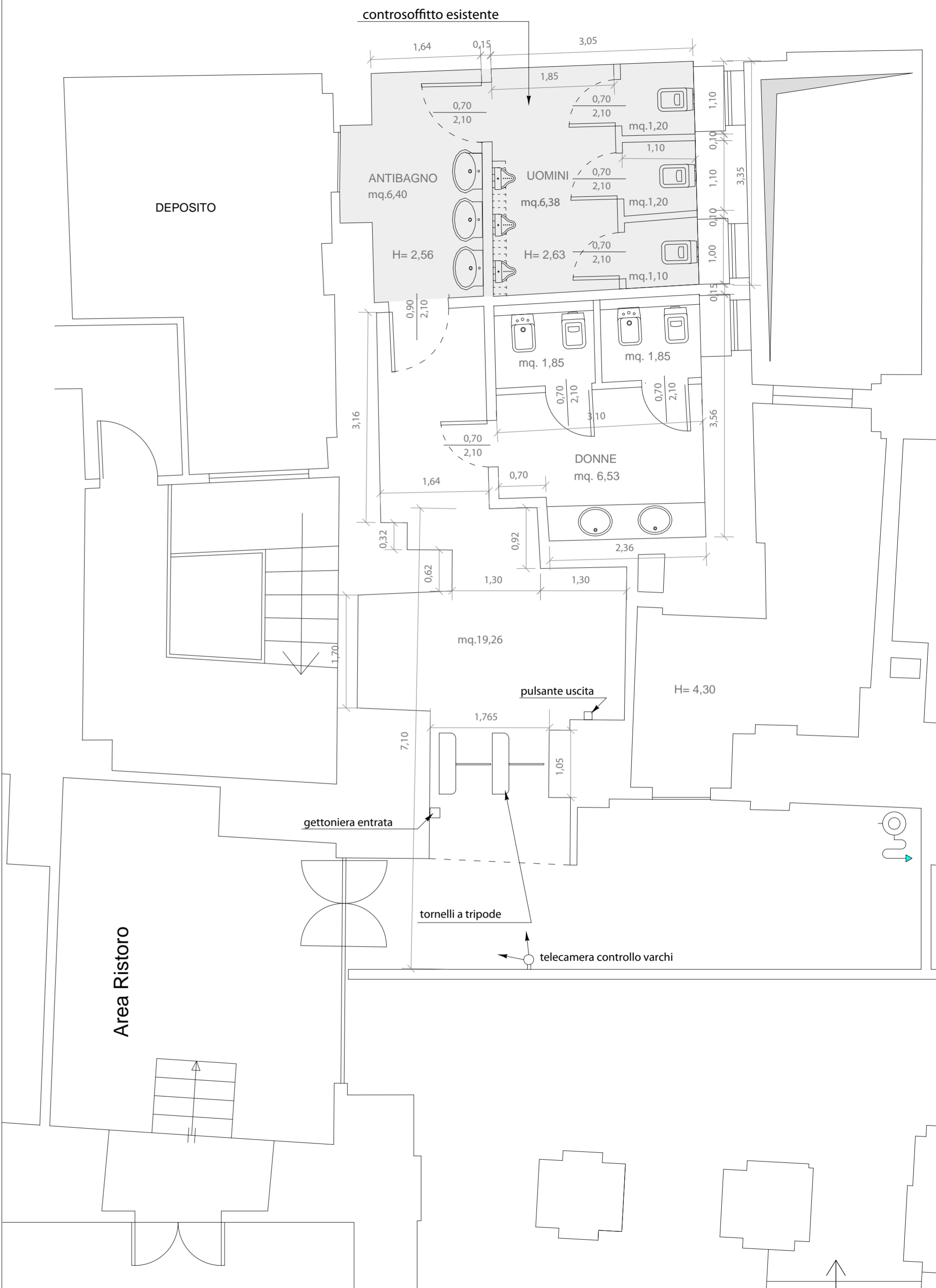
BAGNI INTERRATO - PROGETTO
