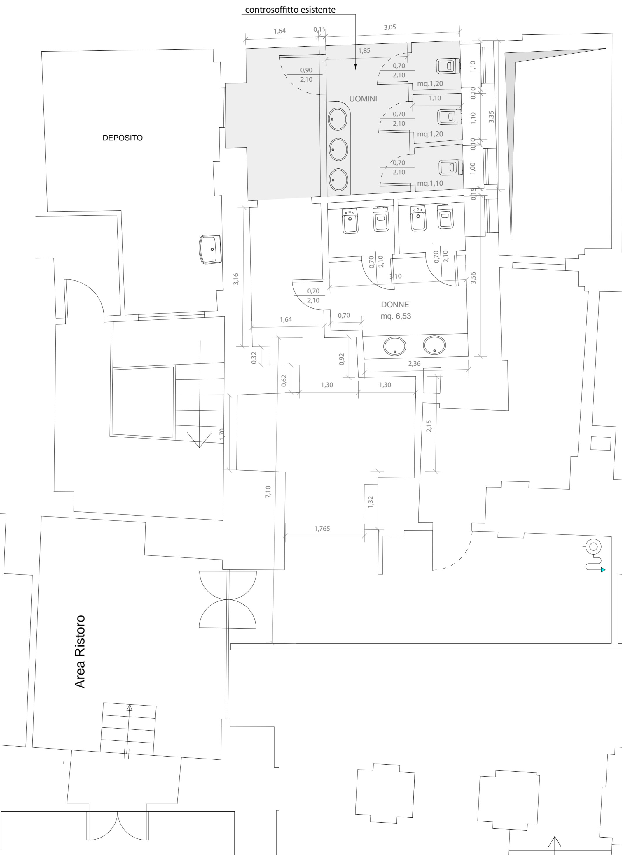
BAGNI INTERRATO - STATO DI FATTO
