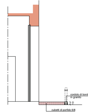
progetto -sezione
