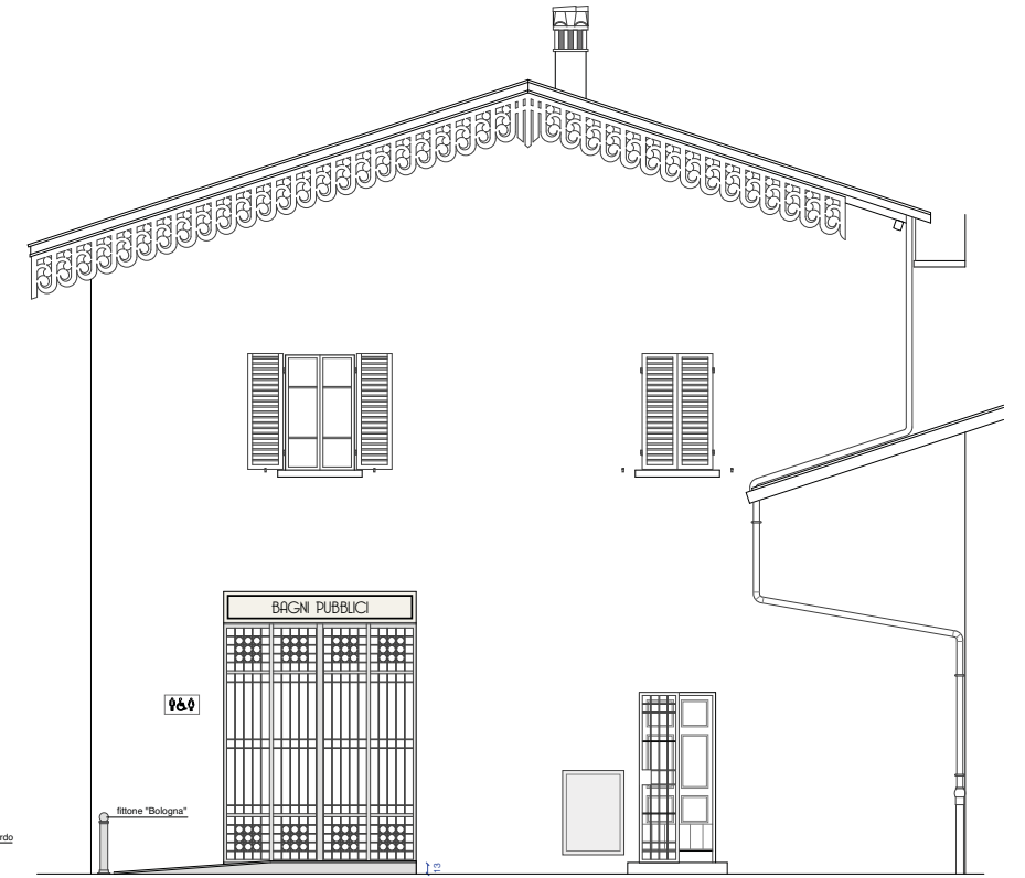
progetto -prospetto
