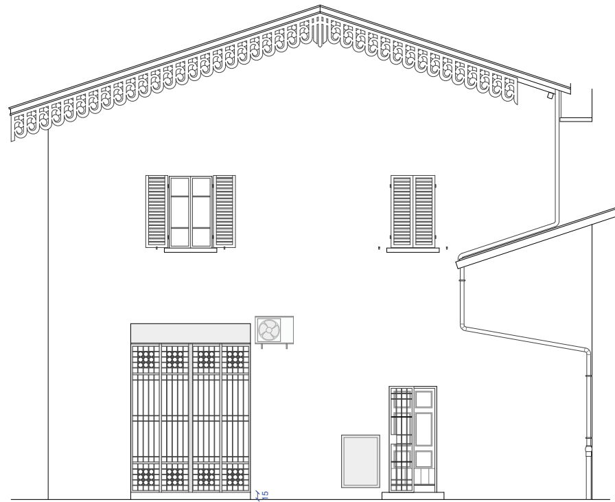
stato di fatto -prospetto
