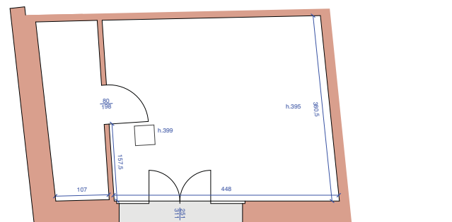
stato di fatto -pianta
