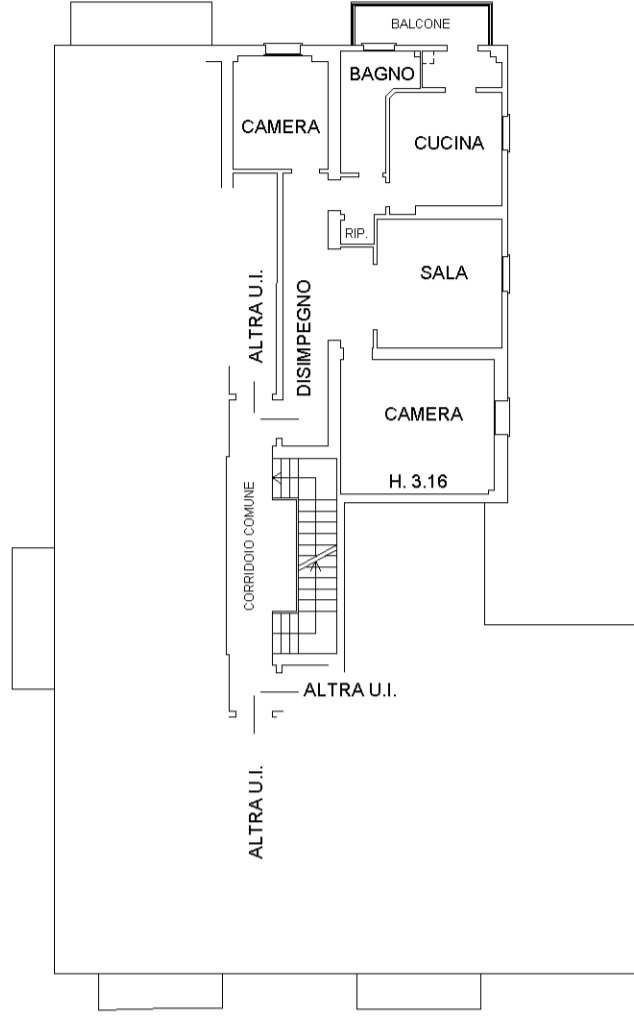
PIANO SECONDO
