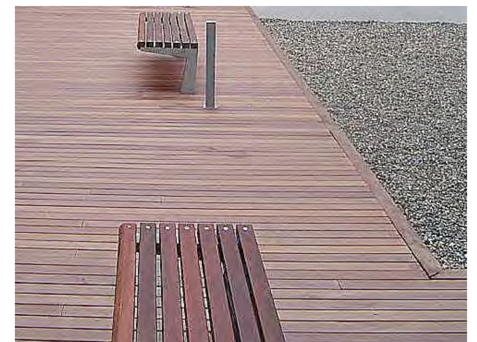
esempio di pavimentazione in doghe di legno di larice posata su struttura con magatelli in legno ancorati al terreno
