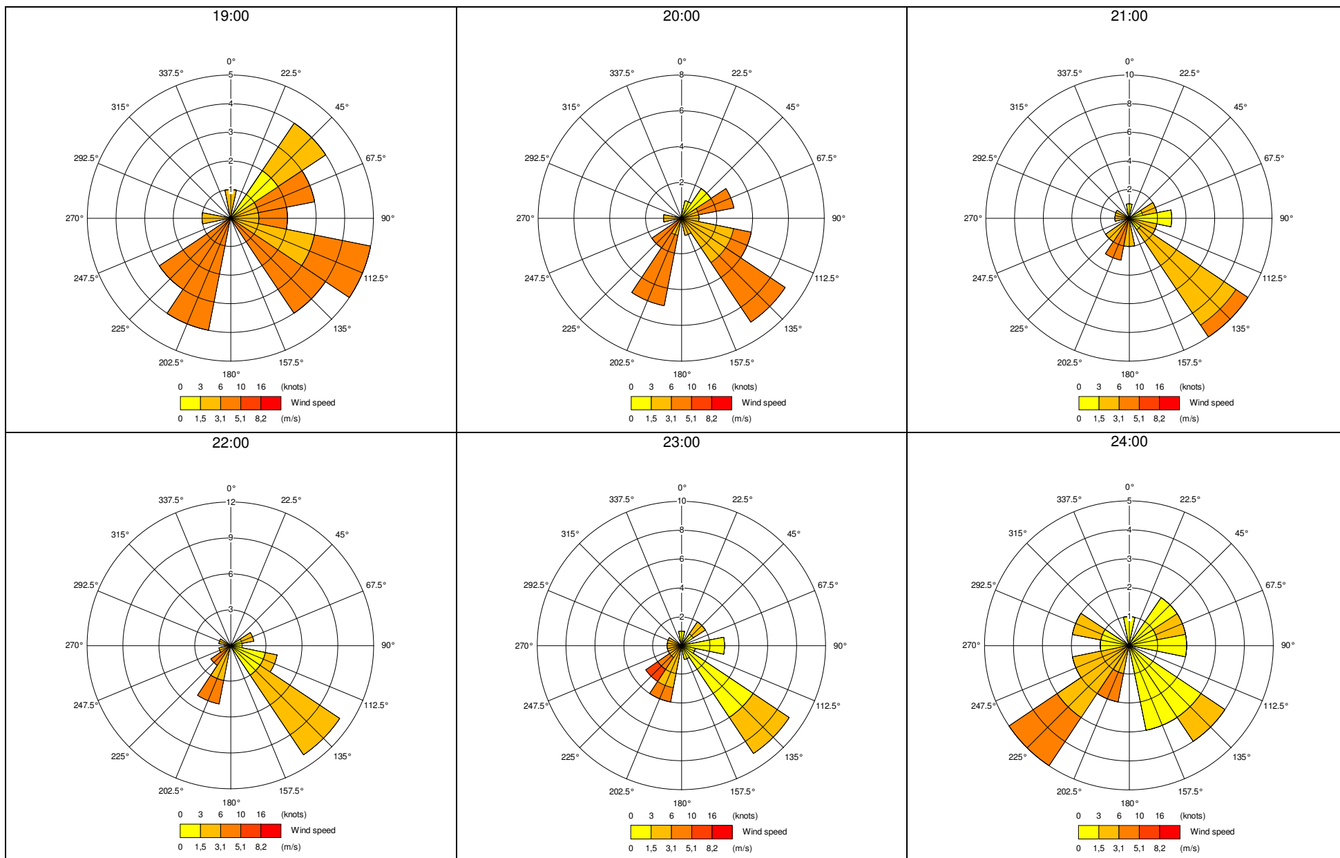
Figura A.3.5 – Profili anemometrici relativi alle singole ore calcolate sul periodo dal 12/7 al 7/8 e registrati nella Postazione A.
