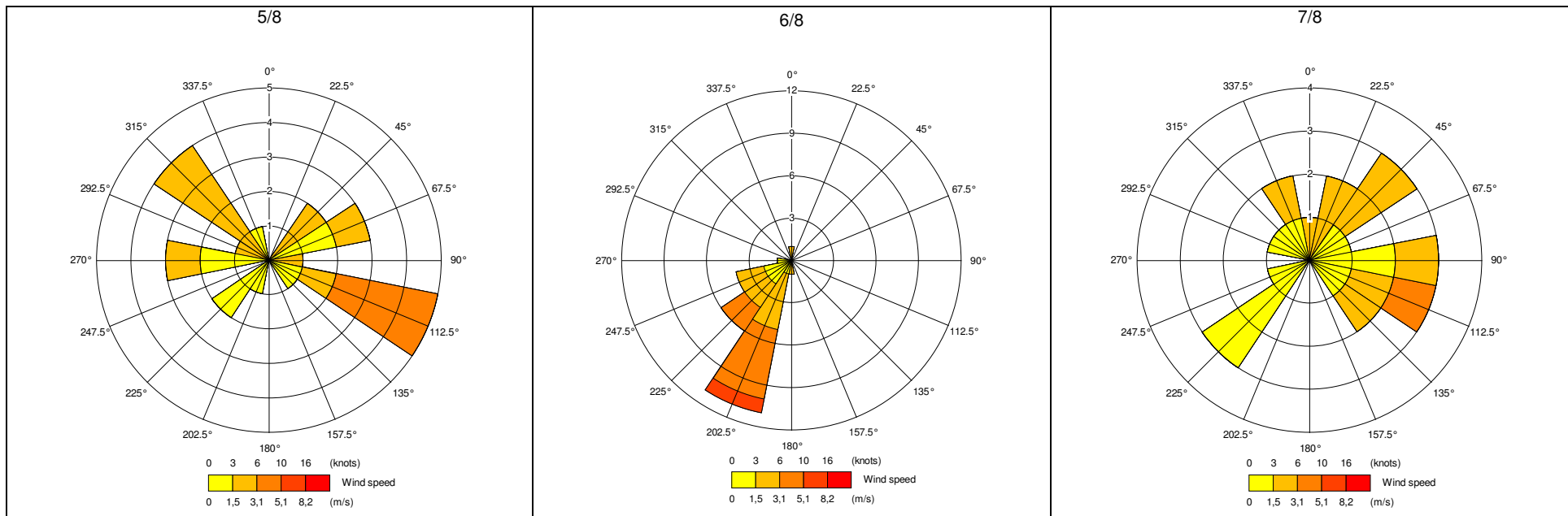
Figura A.3.4 – Profili anemometrici giornalieri del periodo dal 12/7 al 7/8 registrati nella Postazione B.
