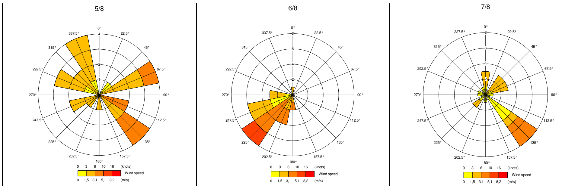
Figura A.3.3 – Profili anemometrici giornalieri del periodo dal 12/7 al 7/8 registrati nella Postazione A.
