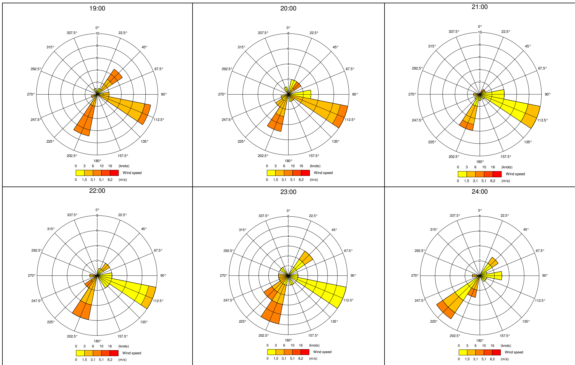
Figura A.3.6 – Profili anemometrici relativi alle singole ore calcolate sul periodo dal 12/7 al 7/8 e registrati nella Postazione B.
