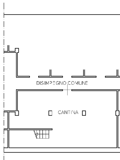
PIANTA PIANO INTERRATO H=2,35
