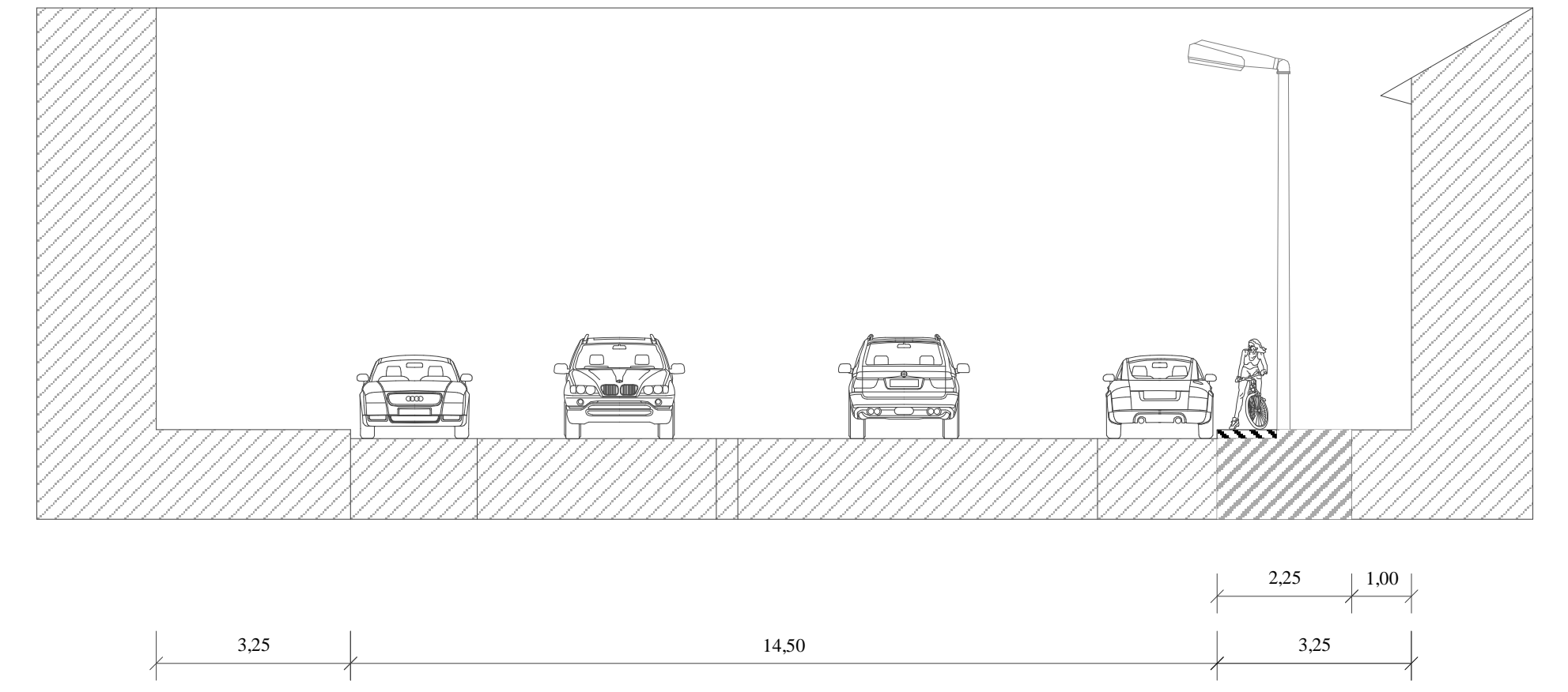
SEZ. CC scala 1:100
