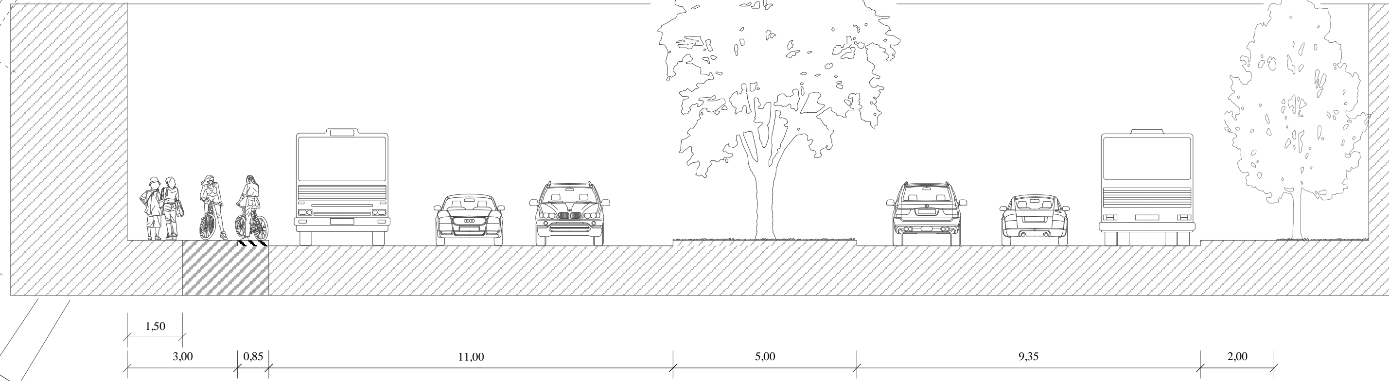
SEZ. AA scala 1:100
