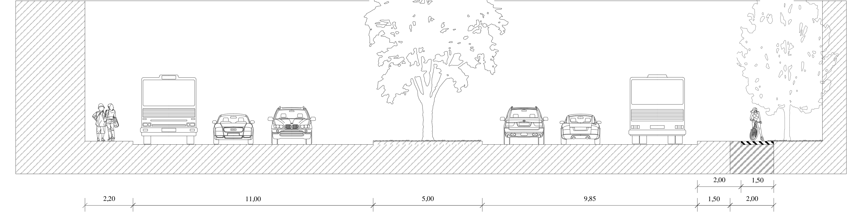
SEZ. BB scala 1:100
